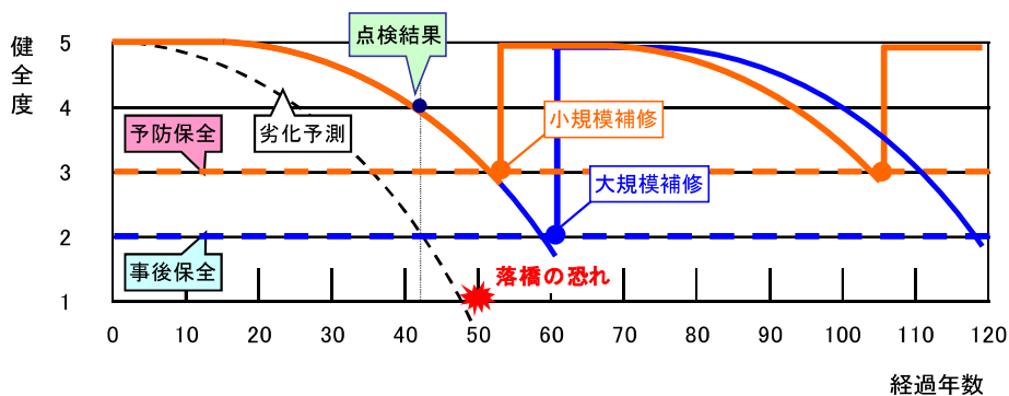
図3. 維持管理シナリオ
