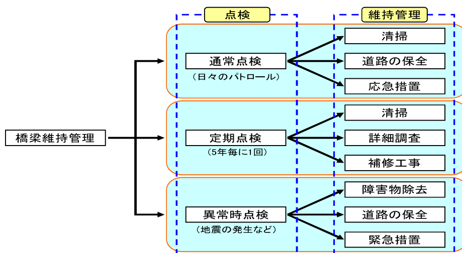
図2. 橋梁の点検および維持管理の体系
